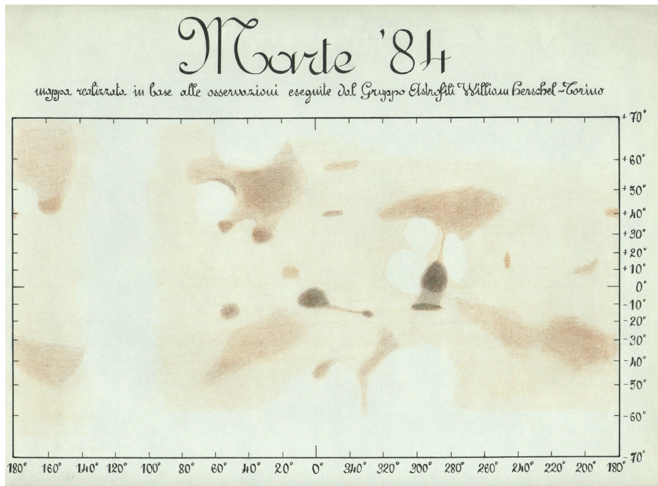
Mappa di Marte nell'opposizione 1984 realizzata con le osservazioni dei soci del G.A.W.H.
