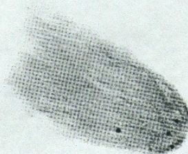
M78 osservata con un rifrattore 120/1800 sotto un cielo di mag. visuale 5
