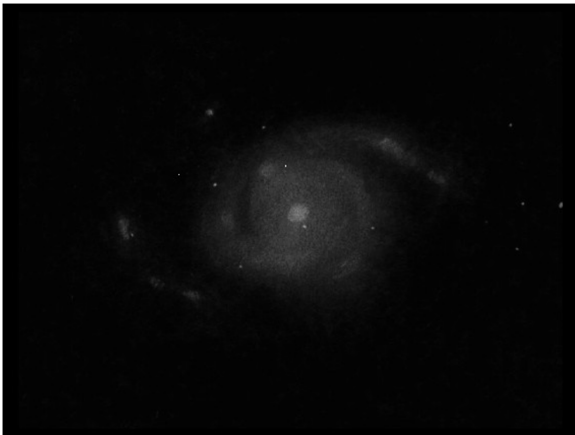
M101 e le sue regioni HII osservata con Newton da 40 cm. Disegno Giancarlo Forno.
