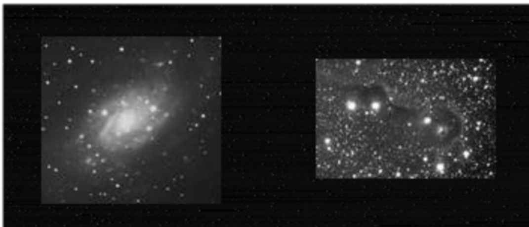
NGC 2403 (Giraffa) e VdB 142 in IC 1396 (Cefeo): immagini CCD riprese da Aldo Proietti.
