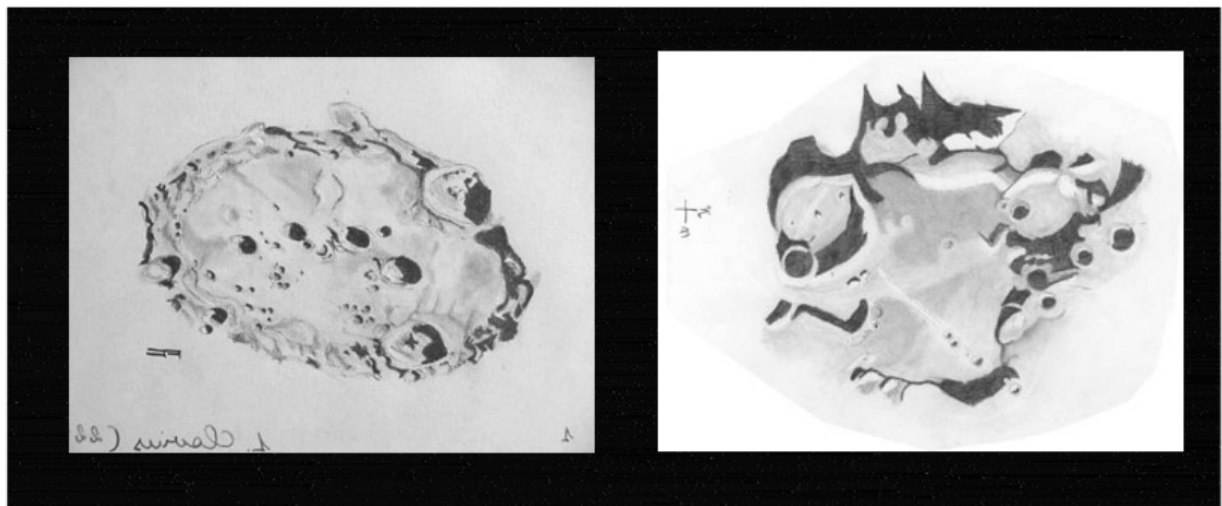
La Luna disegnata da Federico Corno: a sinistra il grande circo Clavio con riflettore 200mm; a destra il cratere Davy e la catena di craterini Davy con rifrattore 102mm.
