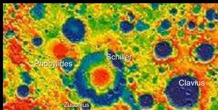
Fig. 8: mappa gravitazionale della sonda GRAIL; in rosso al centro un picco gravitogeno (mascon) in corrispondenza della zona che stiamo studiando
