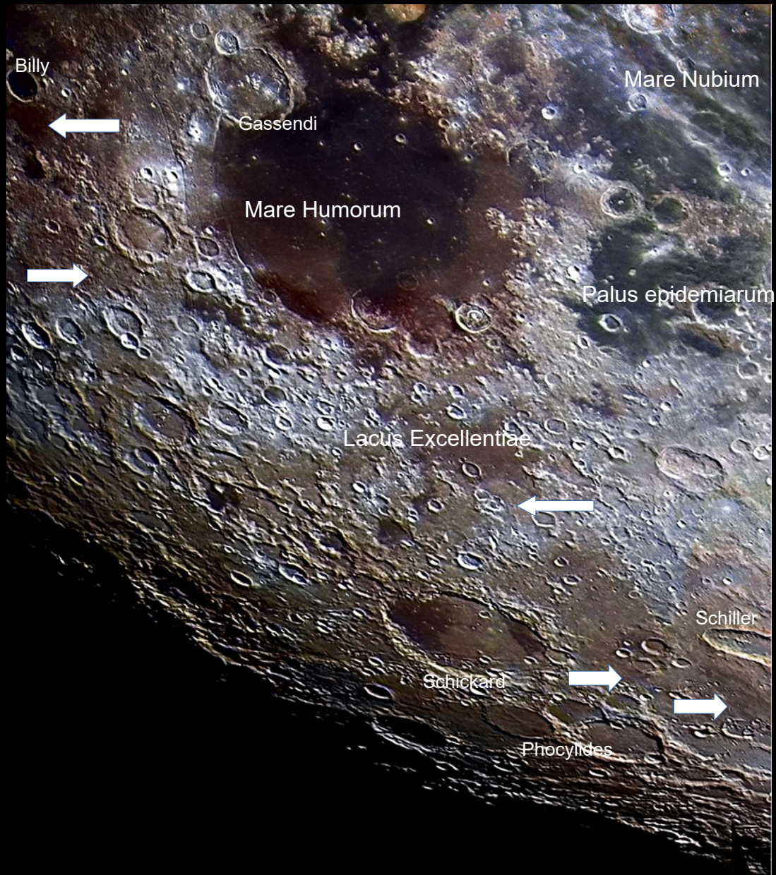
Fig. 4: Immagine selenocromatica dell'area tra Mare Humorum e Schickard, età della luna 13, 34 giorni; le frecce indicano highlands piatte e di maggiore colorito rosso. Mosaico di A. Ferruggia con C8/10 e ASI 224MC
