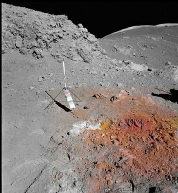
Fig. 3: Immagine di suolo lunare dalla missione Apollo 17; in basso ed a destra area dai colori cangianti (dal giallo al rosso passando per l'arancione) in relazione alle diverse concentrazioni di cristalli di \text{TiO}_2 . Da http://www.psrhawaii.edu/CosmoSparks/Jan19/lunar-orange-glass-beads.html
